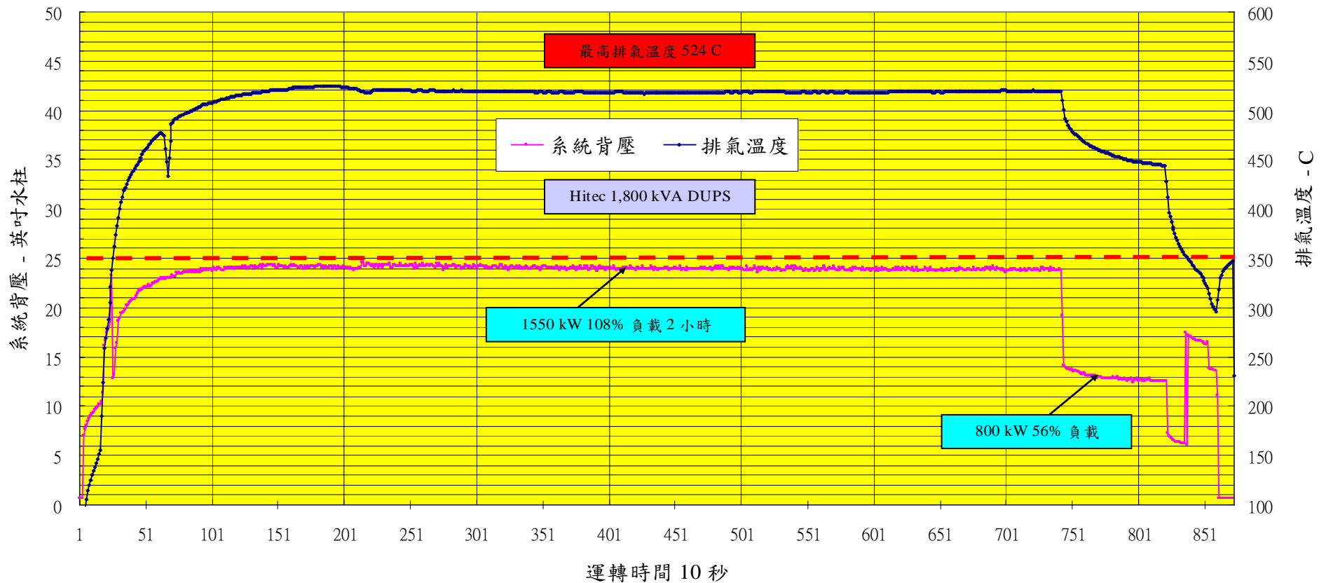
PMOS - 0532 茂德 DUPS 3 超载1,550 kW 温度背压曲线 06 April 2006
