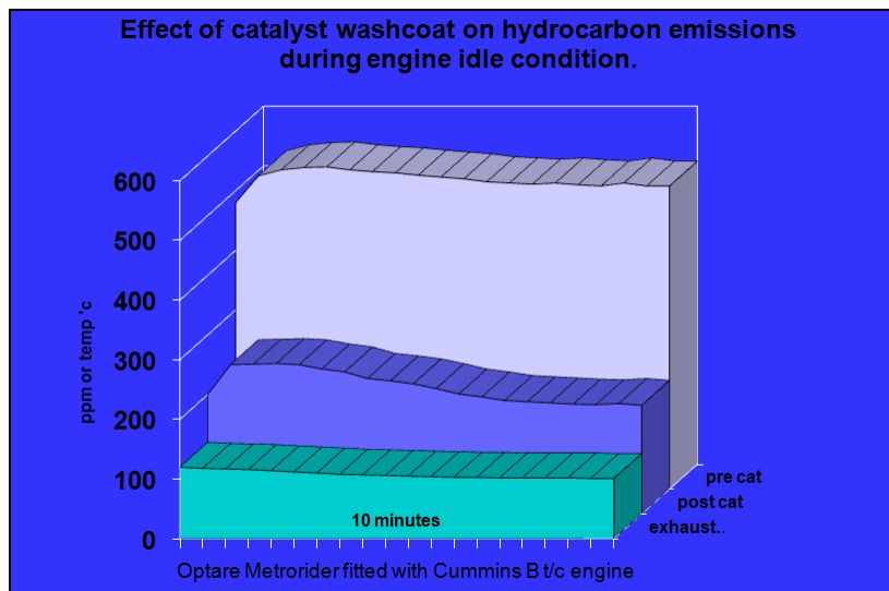
低排氣溫度廢氣-「碳氫化合物」處理效率
