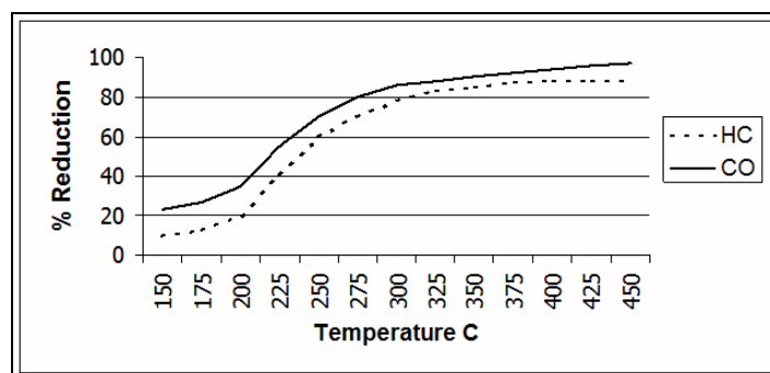
「HC 碳氫化合物」「CO 一氧化碳」處理效率 DZ 型「觸媒轉化器」
