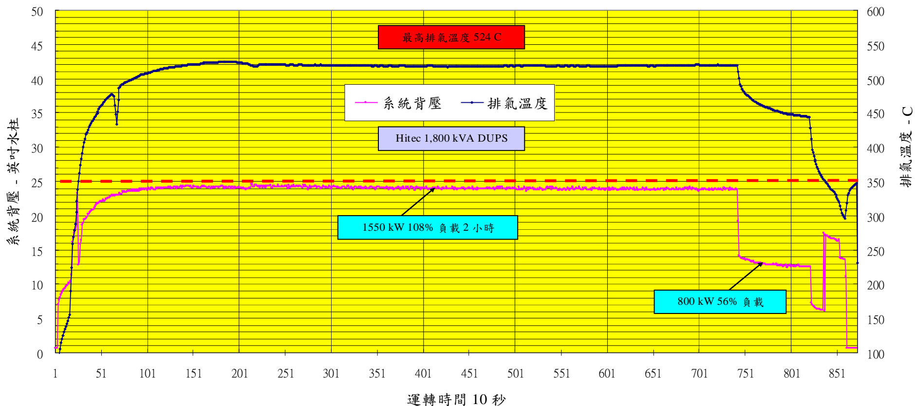
PMOS - 0532 茂德 DUPS 3 超載1,550 kW 溫度背壓曲線 06 April 2006
